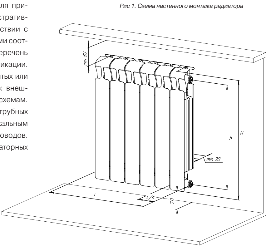
Рис 1. Схема настенного монтажа радиатора
